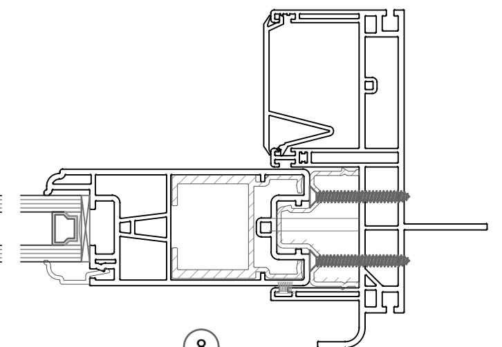
8 Jamb Detail
