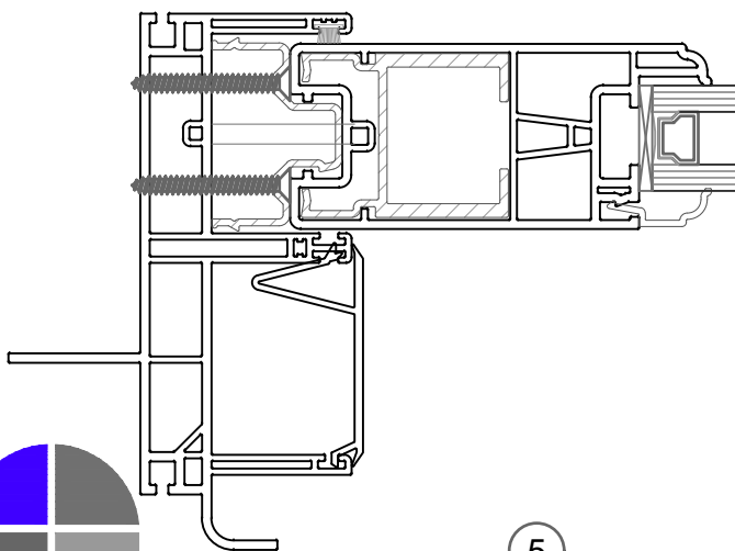
5 Jamb Detail
